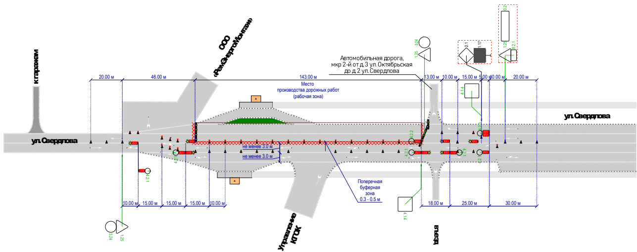
Схема организации дорожного движения и ограждения рабочей зоны при проведении работ на нечётной стороне 4-х полосного участка ремонта.
