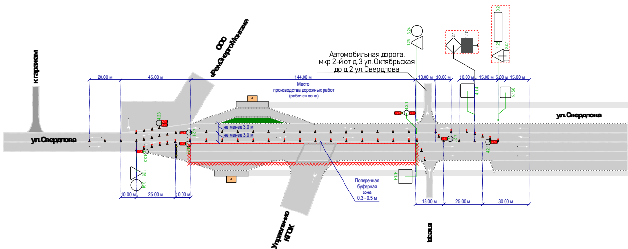
Схема организации дорожного движения и ограждения рабочей зоны при проведении работ на чётной стороне 4-х полосного участка ремонта.
